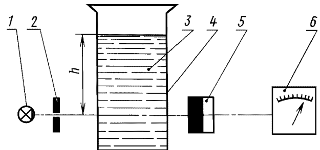
1 — источник света; 2 — диафрагма; 3 — суспензия порошка; 4 — ; 5 — ; 6 — ( )
